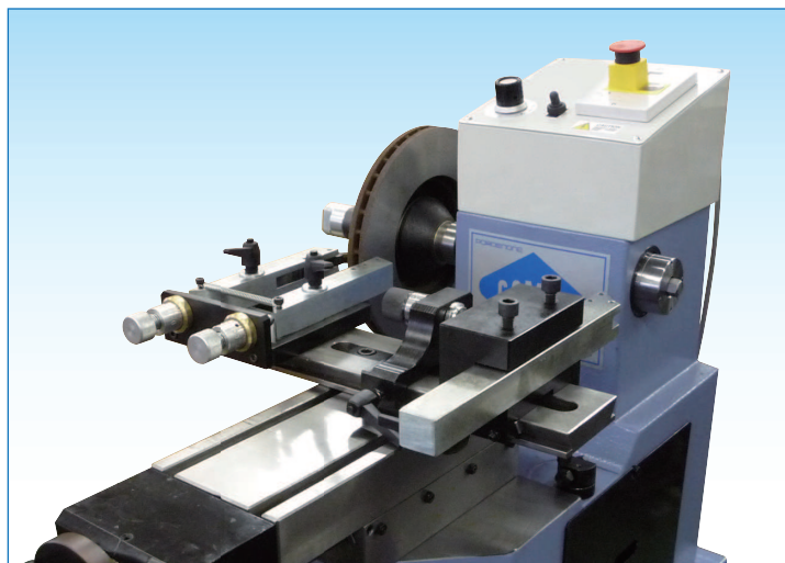
ディスク切削（送り方向はスピンドルに対して垂直）
